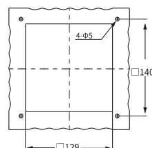
安裝孔 VFU04A
