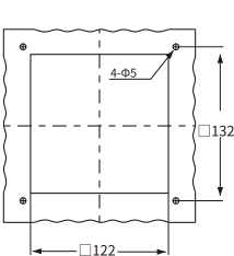
安裝孔 VFU03
