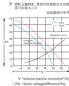
功率特性曲線
