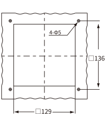
安裝孔 VFU04B
