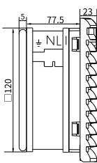
風機及過濾器 VFU06B
