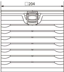
風機及過濾器 VFU06B
