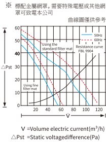
功率特性曲線
