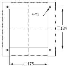
安裝孔 VFU06B
