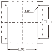
安裝孔 VFU02
