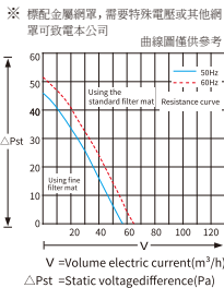
功率特性曲線
