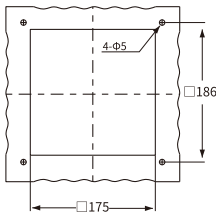
安裝孔 VFU06A
