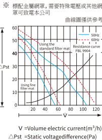
功率特性曲線
