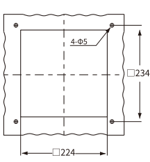
安裝孔
